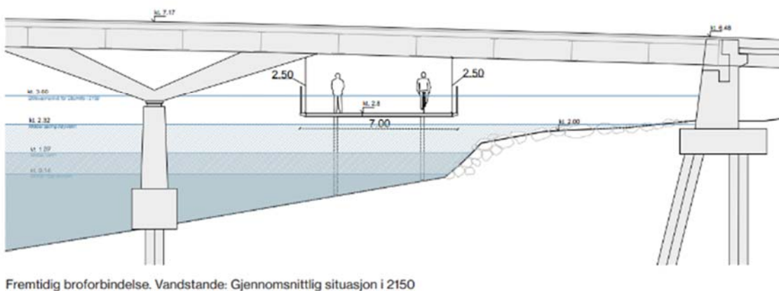
Forslag til klimasikker gang-/sykkelbru under Pirbrua.
